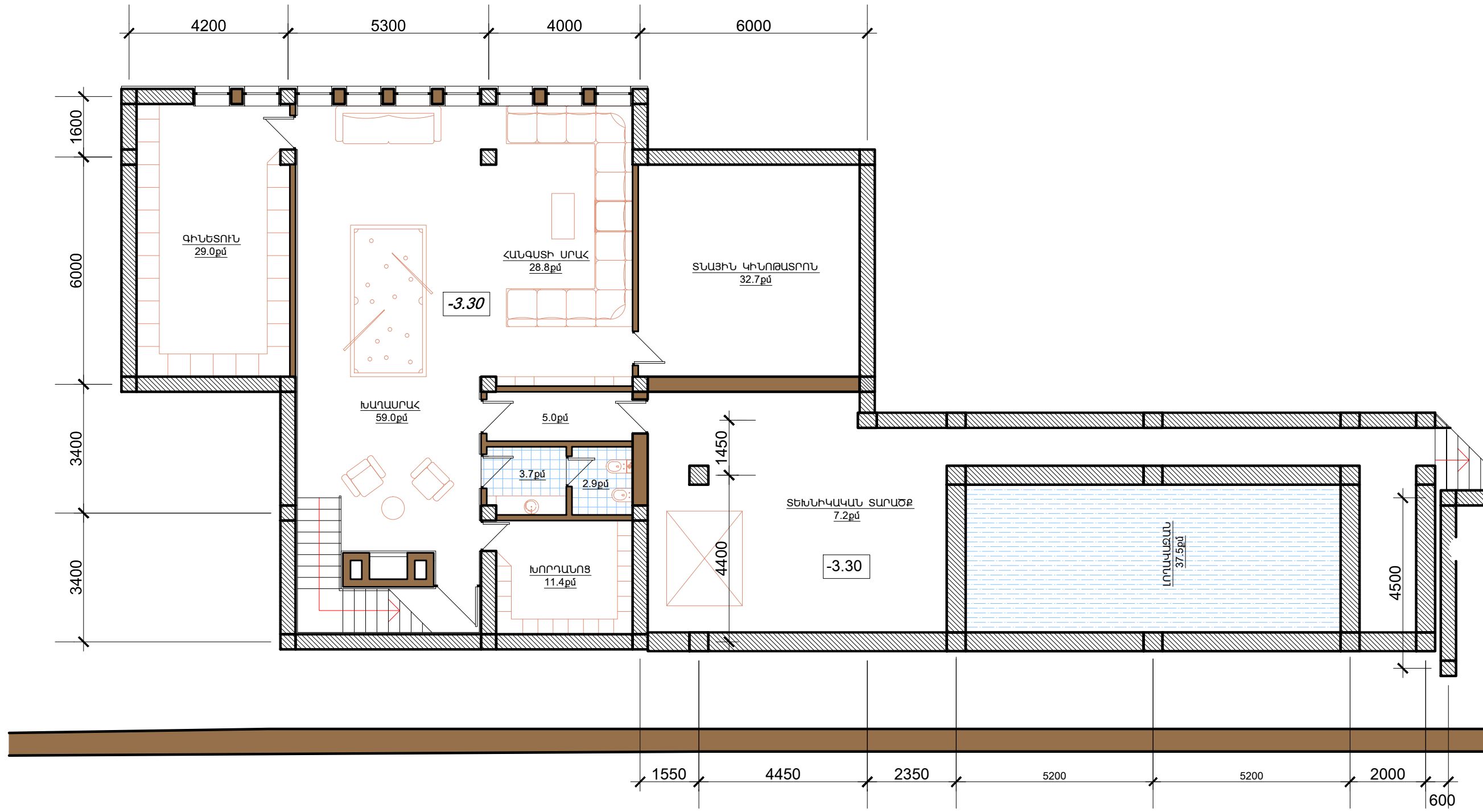
ՆԿՈՒԱՅԻՆ ԶԱՐԿԻ ԶԱՏԱԿԱԳԻԾ (ԿԱՅԱՎՈՐՈՒՄՈՎ) -3.30 ՆԻՇՈՒՄ Մ-1:100
